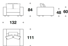
ORT (POL) POLTRONA / ARMCHAIR 132x111x84H. - H.A.60 - H.S.48 cm 52x43 2/3x33H. - H.A.23 2/3 - H.S.19 "
